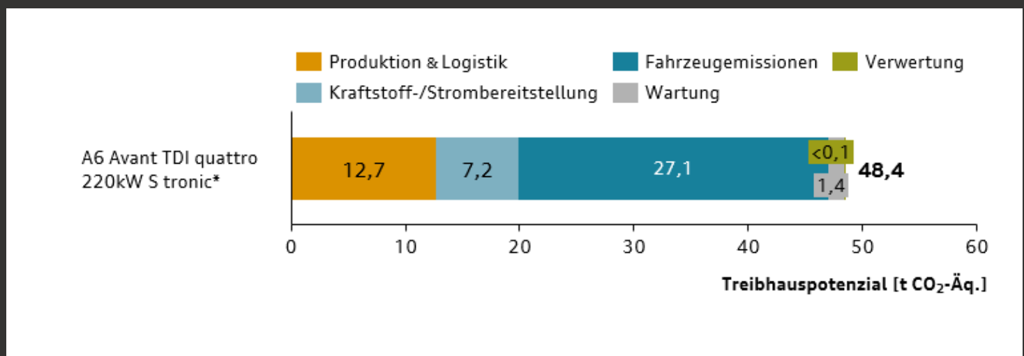
Abbildung 2: Treibhauspotenzial des Audi A6 Avant TDI quattro 220kW S tronic* über den gesamten Lebenszyklus
