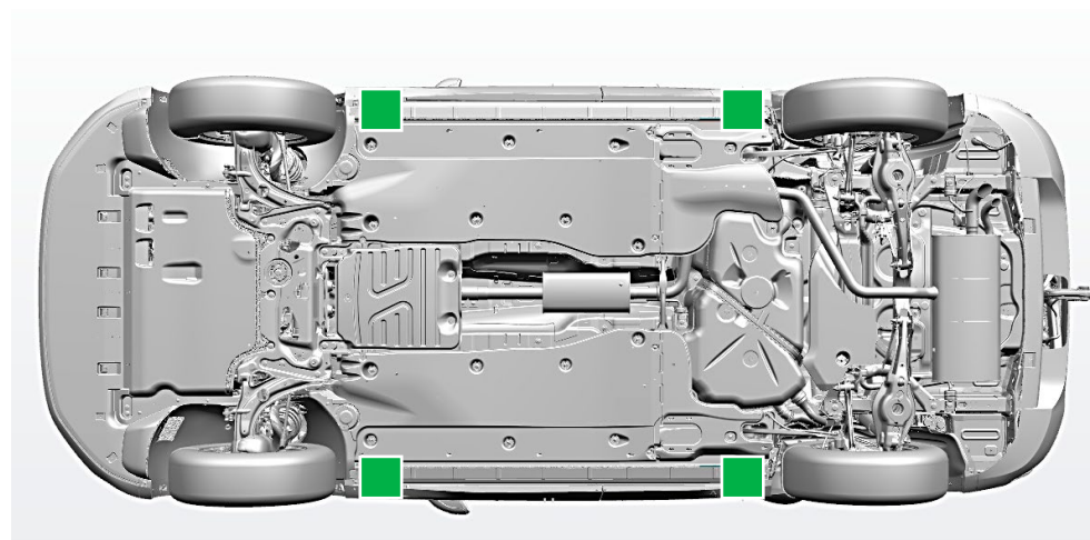
Geeignete Hebe Punkte am Beispiel Audi A5
