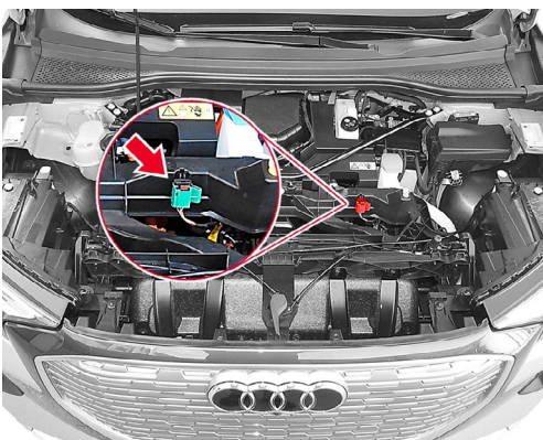
Trennstelle im Motorraum Audi Q4 e-tron
