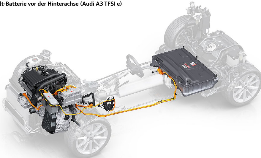
Hochvolt-Batterie vor der Hinterachse (Audi A3 TFSI e)
