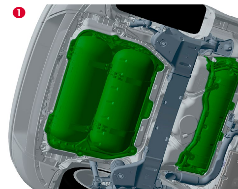
1 Tankabdeckungen am Unterboden entfernen. Die Tankabdeckungen sind in dieser Abbildung grün gekennzeichnet.
