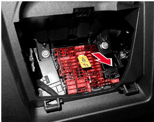
Rettungstrennstelle Sicherungsträger
