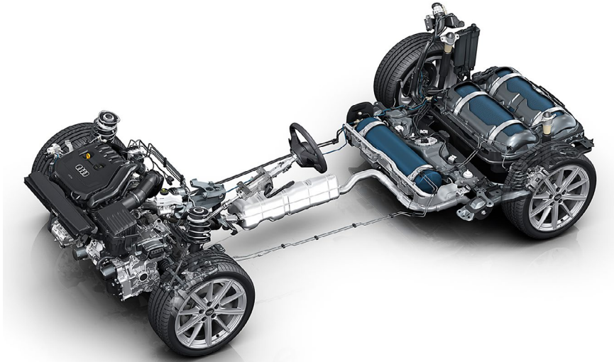
Audi A3 g-tron mit 3 Gastanks
