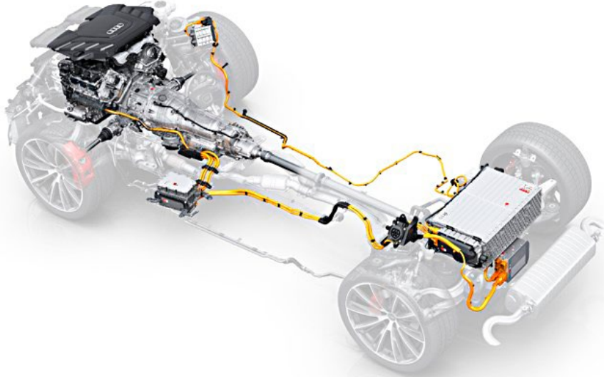
Hochvolt-Batterie im Fahrzeugheck (Audi Q8 TFSI e)
