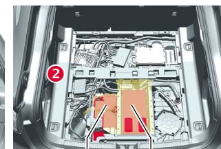
Batterie 12 V Batterie 48 V
