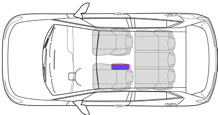
Airbag central à l'avant côté tunnel
