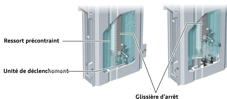
Dispositif de protection en cas de retournement non déclenché
