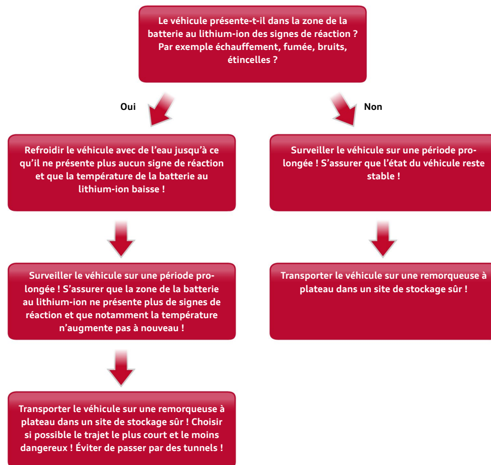
Diagramme de déroulement du remorquage des véhicules électriques
