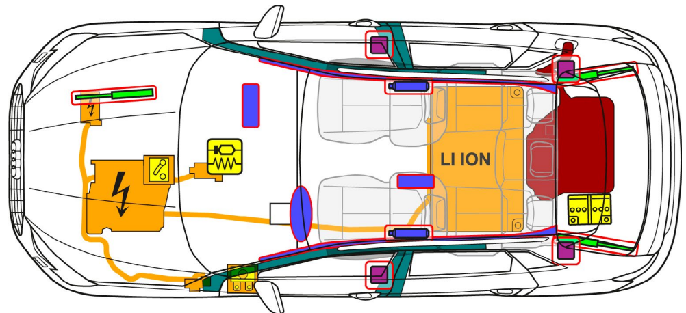
Fiche de secours Audi A3 TFSI e
