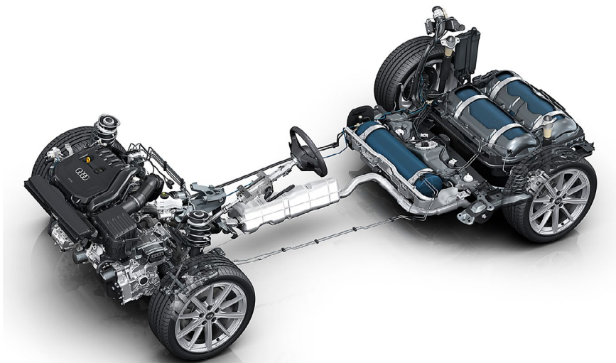
Audi A3 g-tron avec 3 réservoirs à gaz
