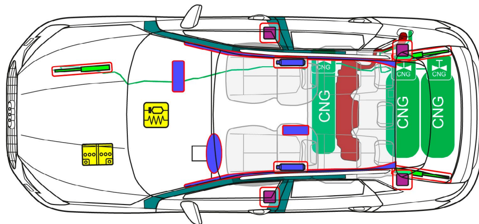
Fiche de secours Audi A3 g-tron (selon ISO 17840)
