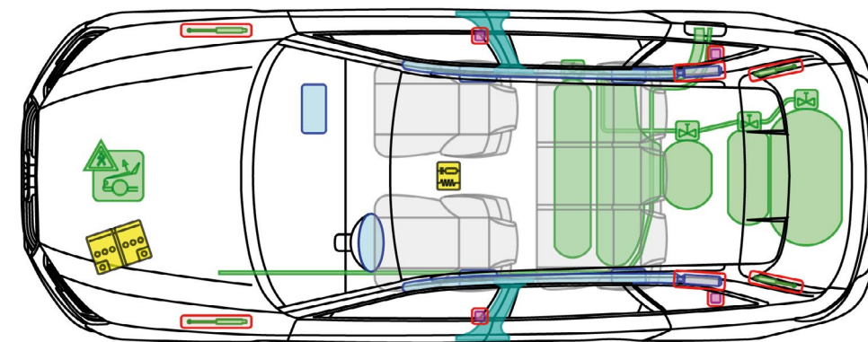
Fiche de secours Audi A4 g-tron (ne correspond pas à la norme ISO 17840 actuelle)
