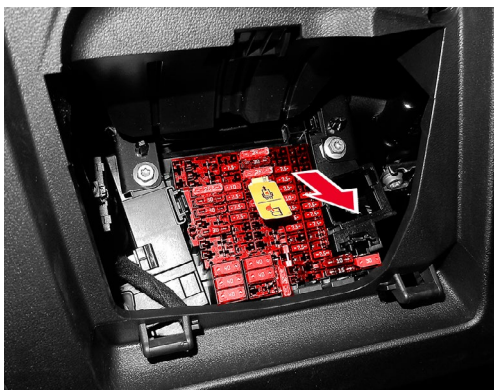
Dispositif de coupure d'urgence sur le porte-fusibles
