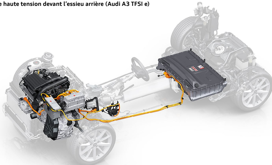
Batterie haute tension devant l'essieu arrière (Audi A3 TFSI e)
