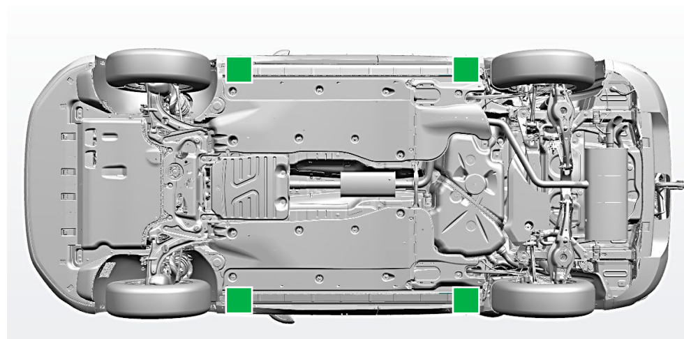
Puntos de elevación adecuados en el Audi A5 a modo de ejemplo
