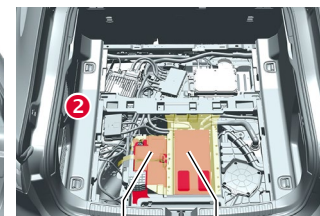
Batería de 12 voltios Batería de 48 voltios
