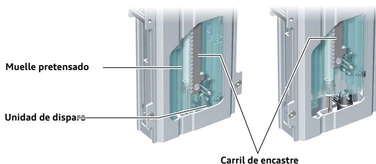
Protección antivuelco sin disparar
