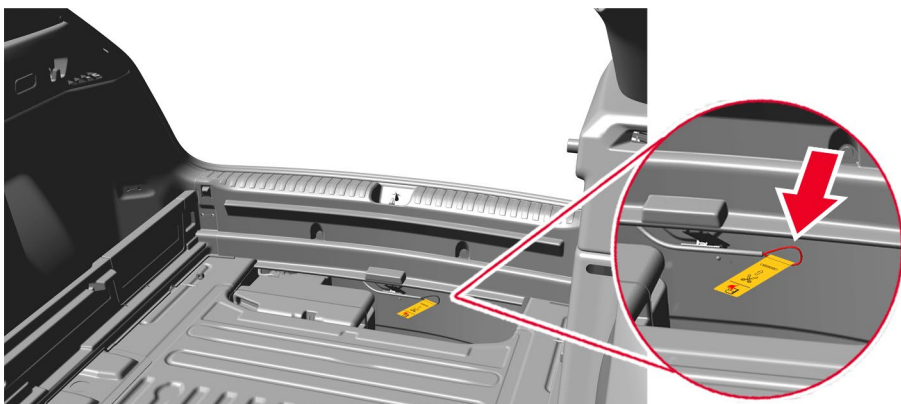
Punto de corte en el maletero del Q4 e-tron debajo del suelo, en el borde. La banderita amarilla señala el punto de corte.
