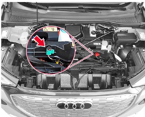
Punto de corte en el vano motor del Audi Q4 e-tron
