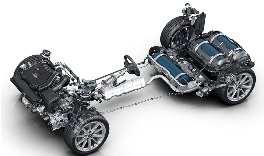
Audi A3 g-tron con 3 depósitos de gas
