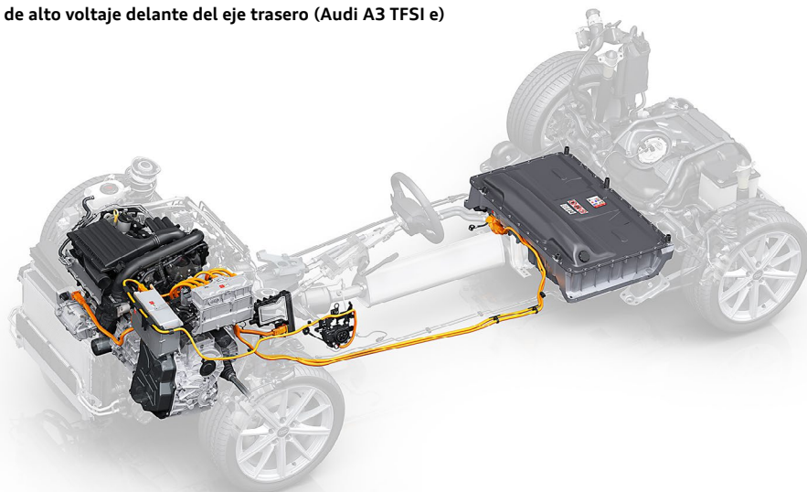
Batería de alto voltaje delante del eje trasero (Audi A3 TFSI e)
