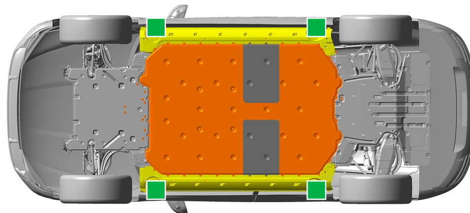
Puntos de elevación adecuados en el Audi e-tron GT a modo de ejemplo
