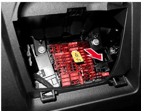
Punto de corte para rescate en el portafusibles
