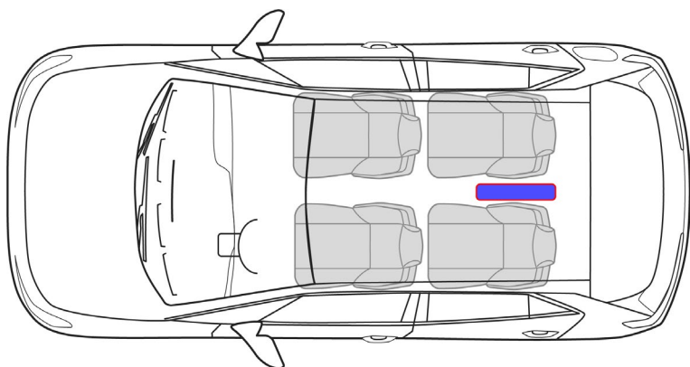
Airbag central trasero en el Audi A8 L de cuatro plazas
